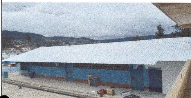
Foto 1: Sustitución de lámina por lámina troquelada aluzinc calibre 26, en dos aulas del módulo 1 y dirección del establecimiento.
